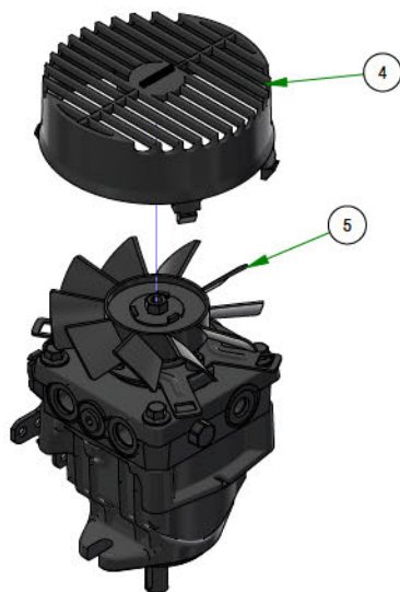
050-3001-00 & 050-3003-00 PUMP ASSEMBLIES
